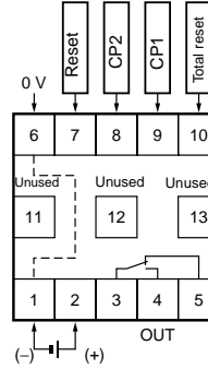
H7CX-AD/-A4D 1-stage Contact Output
