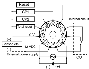
H7CX-A11/-A114/-A11D1/-A114D1 1-stage Contact Output
