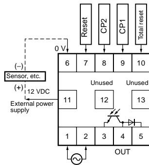
H7CX-AS/-A4S 1-stage Transistor Output
