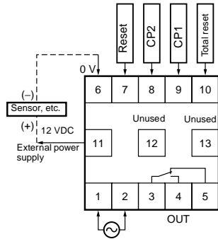
H7CX-A/-A4 1-stage Contact Output
