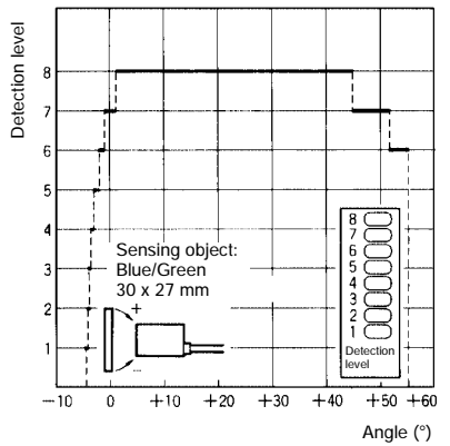
E3MC-(M)Aj j (Y Direction)
