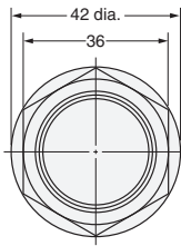
Fig. 31: E2E-X20MD1-M1GJ
