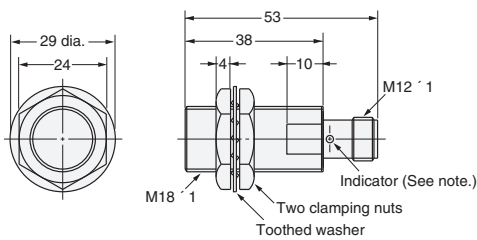
Fig. 20: E2E-X7D□-M1(G)/E2E-X5E□-M1/F□-M1 E2E-X5Y□-M1
