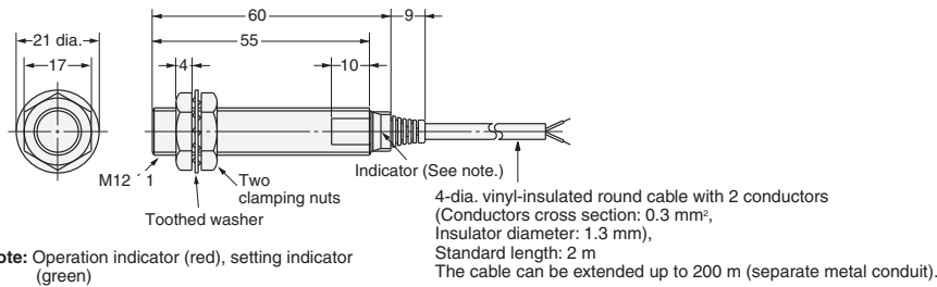
Fig. 10: E2E-X7D□-N/ E2E-X5E□/F□ E2E-X5Y□/E2E-X7T1
