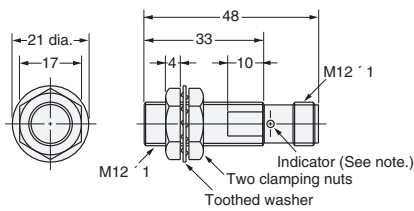
Fig. 16: E2E-X3D□-M1(G) E2E-X2E□-M1/F□-M1
