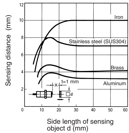
E2E2-X10C/B E2E2-X10Y
