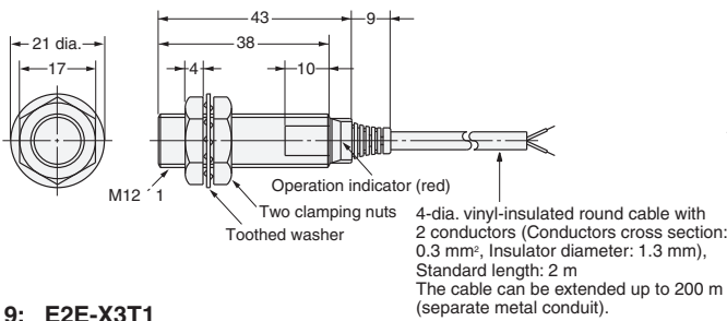
Fig. 9: E2E-X3T1
