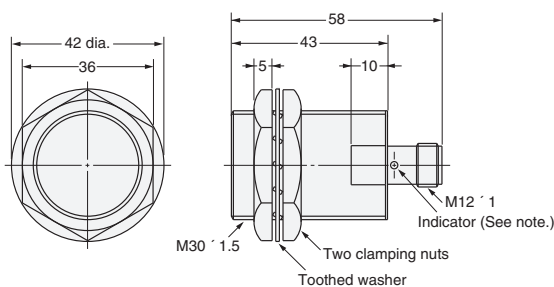
Fig. 22: E2E-X10D□-M1(G)/E2E-X10E□-M1/F□-M1 E2E-X10Y□-M1
