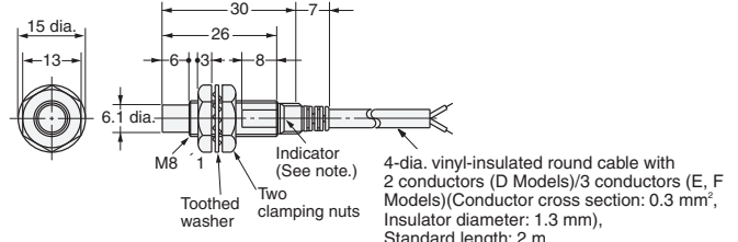
Fig. 2: E2E-X4MD□ E2E-X2ME□/F□
