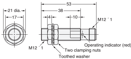
Fig. 18: E2E-X2Y□-M1
