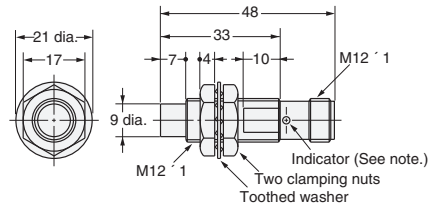
Fig. 17: E2E-X8MD□-M1(G) E2E-X5ME□-M1/F□-M1
