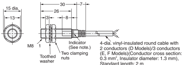
Fig. 1: E2E-X2D□-N E2E-X1R5E□/F□
