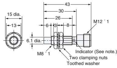
Fig. 15: E2E-X4MD□-M1(G) E2E-X2ME□-M1/F□-M1
