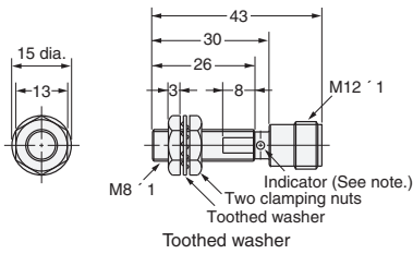
Fig. 14: E2E-X2D□-M1(G) E2E-X1R5E□-M1/F□-M1
