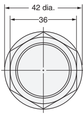
Fig. 30: E2E-X10D1-M1GJ E2E-X10D1-M1J-T
