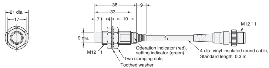
Fig. 28: E2E-X7D1-M1GJ E2E-X7D1-M1J-T
