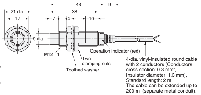
Fig. 8: E2E-X5MY□
