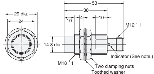
Fig. 21: E2E-X14MD□-M1(G)/E2E-X10ME□-M1/F□-M1 E2E-X10MY□-M1
