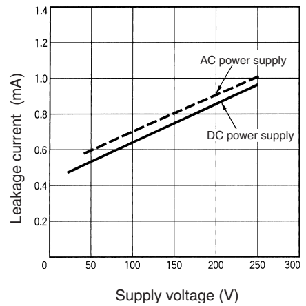
E2E-X□T1 DC/AC
