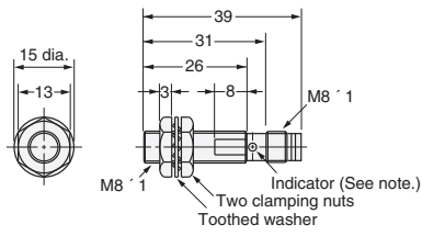
Fig. 24: E2E-X2D□-M3G/E2E-X1R5E□-M3/F□-M3
