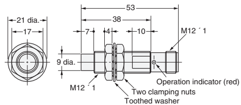
Fig. 19: E2E-X5MY□-M1
