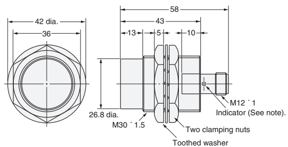
Fig. 23: E2E-X20MD□-M1(G)/E2E-X18ME□-M1/F□-M1 E2E-X18MY□-M1
