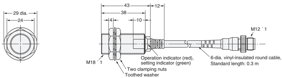
Fig. 28: E2E-X7D1-M1GJ E2E-X7D1-M1J-T
