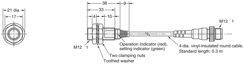
Fig. 26: E2E-X3D1-M1GJ E2E-X3D1-M1J-T
