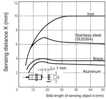
E2E-X10ME□/F□ E2E-X10MY
