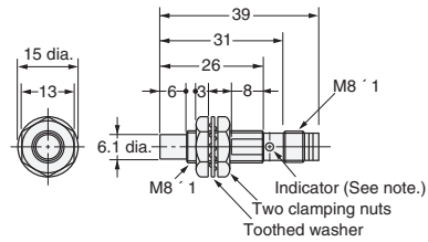
Fig. 25: E2E-X4MD□-M3G/E2E-X2ME□-M3/F□-M3
